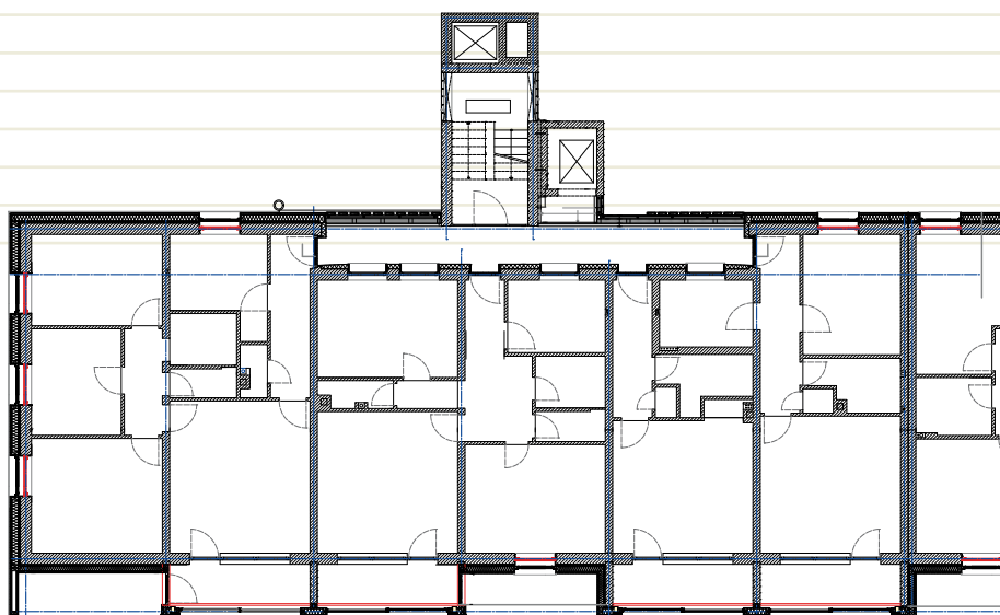
Grundriss
